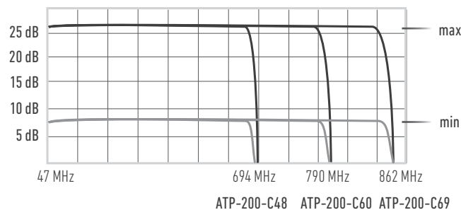
Gráficas de regulación de ganancia
